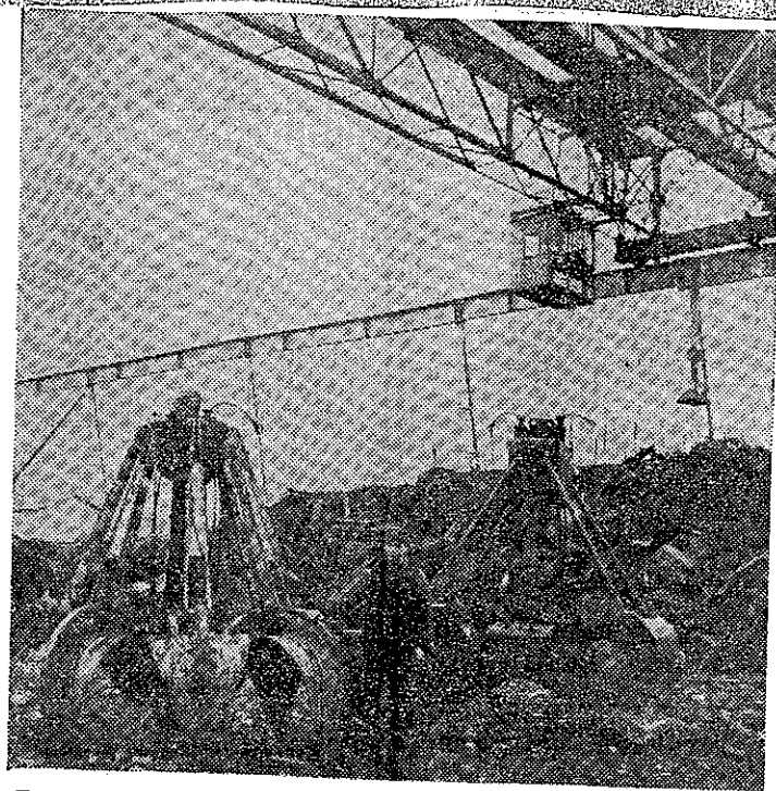
T. v. ses "polypen" och t. h., över skrothögen, svävar magneten
