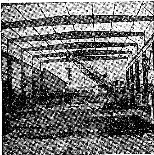
Maskinkranen i arbete med takstolarna
