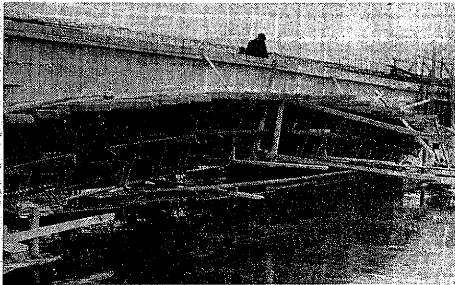
SL-balkarna, som syns under trästativet, underlättar i hög grad brobyggandet därför att de gör på- ningen onödig
