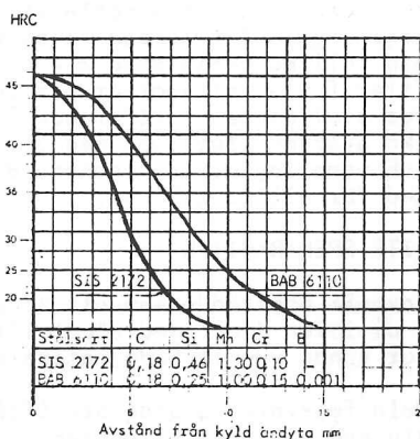
Bild 2. Resultat från jominyprov med SIS 2172 och BAB 6110.
