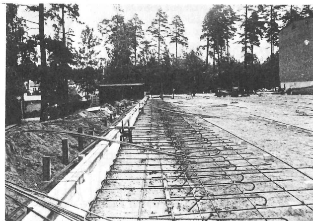
Armering av grundplatta sett mot Älvkullevägen. (79-06-09)
